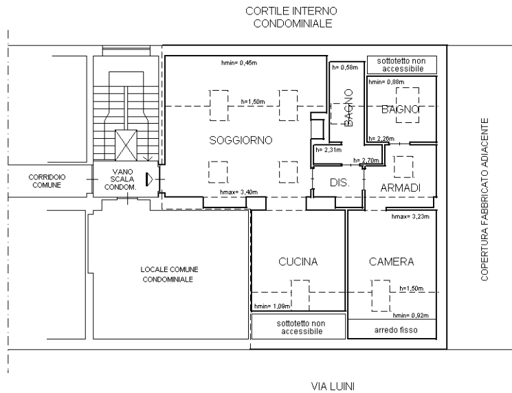
PIANTA PIANO QUARTO (5° f.t.) - hm=2,05m
